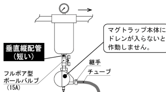
ドレン出口がチューブの場合
