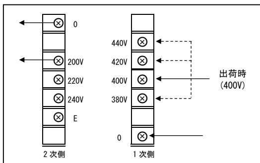
トランス端子台図
